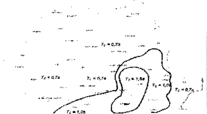
Zonarea teritoriului României, perioadă de revenire (Tc), TC a spectrului de răspuns
